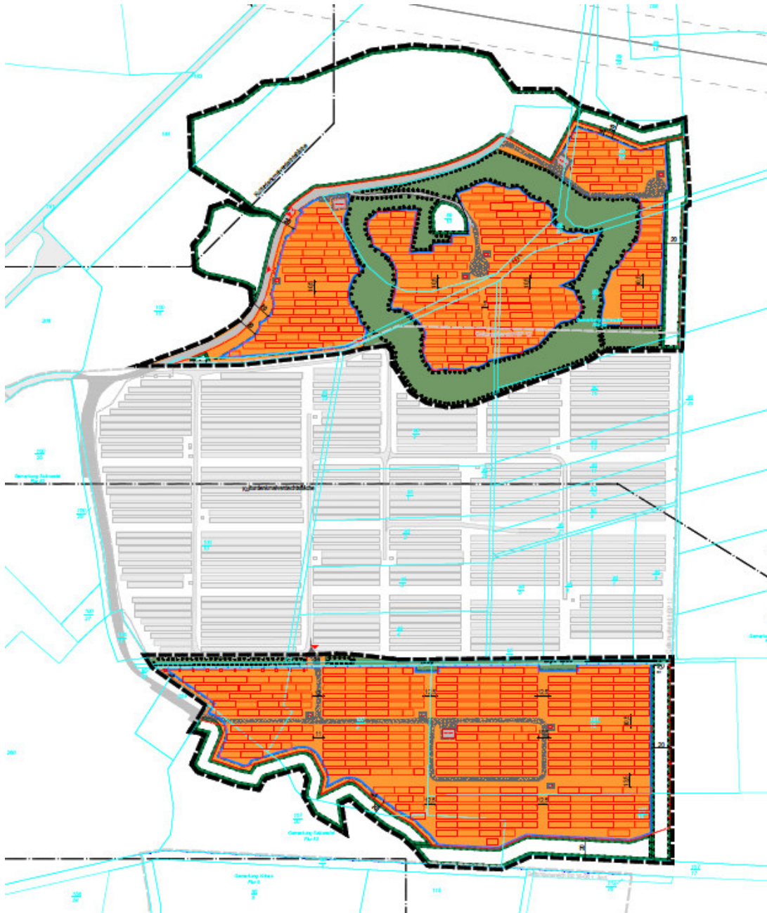
Abbildung 9: Ausschnitt aus dem Vorhaben- und Erschließungsplan, Stand 08.11.2022 ohne Maßstab. Der Plan ist verbindlicher Bestandteil des vorhabenbezogenen Bebauungsplans. Er kann aber geändert werden, soweit er den Festsetzungen des B-Plans nicht widerspricht.
